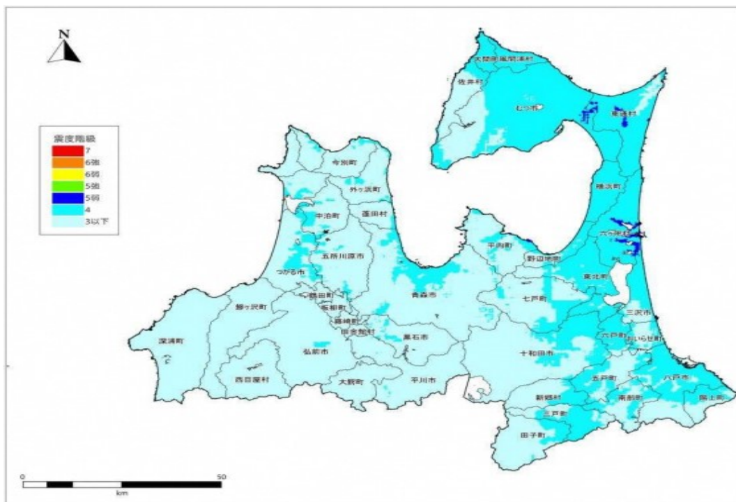
(2) 千島海溝（十勝・根室沖）モデル（マグニチュード9.3）
