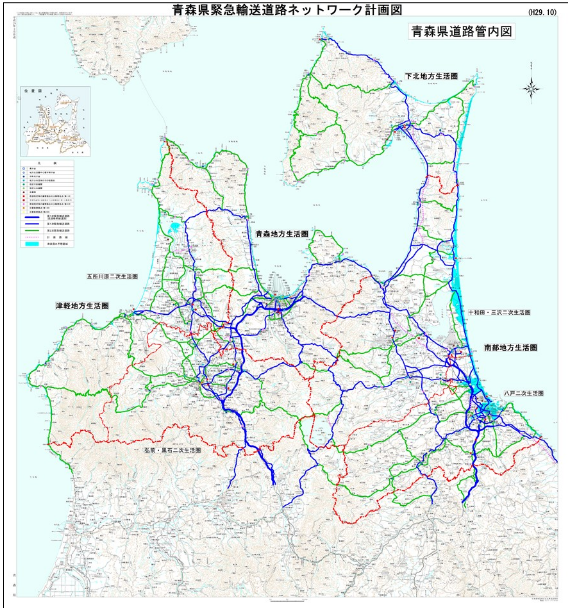
資料 2 青森県緊急輸送道路ネットワーク計画図（県土整備部道路課より）
