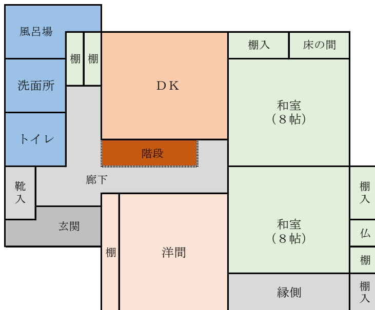
(1階)
